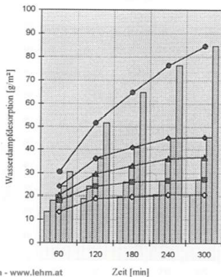
Vergleich Desorption der 1 cm Probekörper
