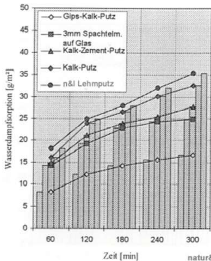
Vergleich Absorption der 1 cm Probekörper
